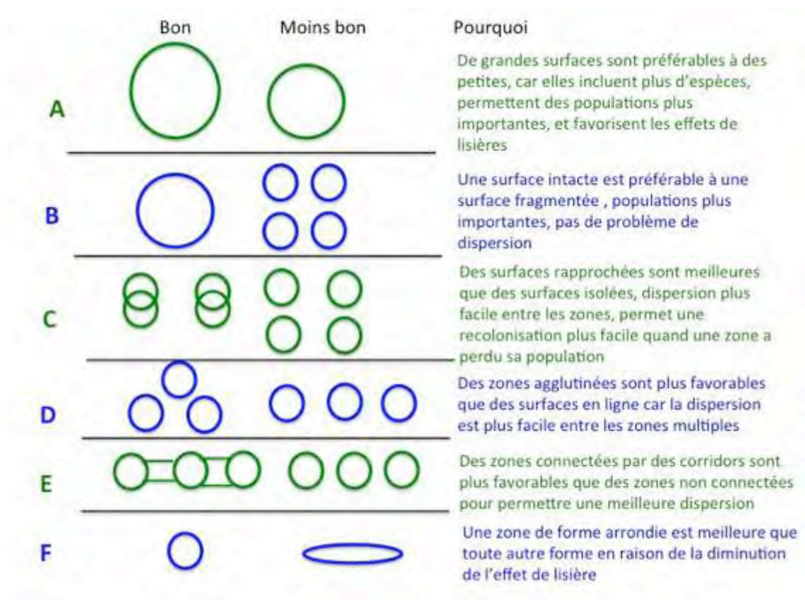
Représentation schématique de la théorie du SL
