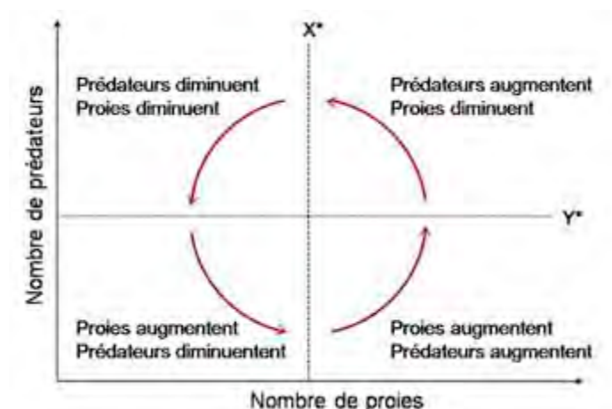
Espaces des phases du modèle de Lotka-Volterra et évolution de l'abondance des proies et des prédateurs.
