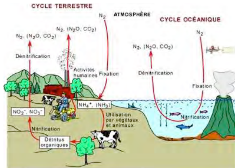
Représentation schématique du cycle de l'azote
